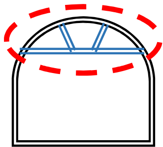
タイバーによるハウス補強
